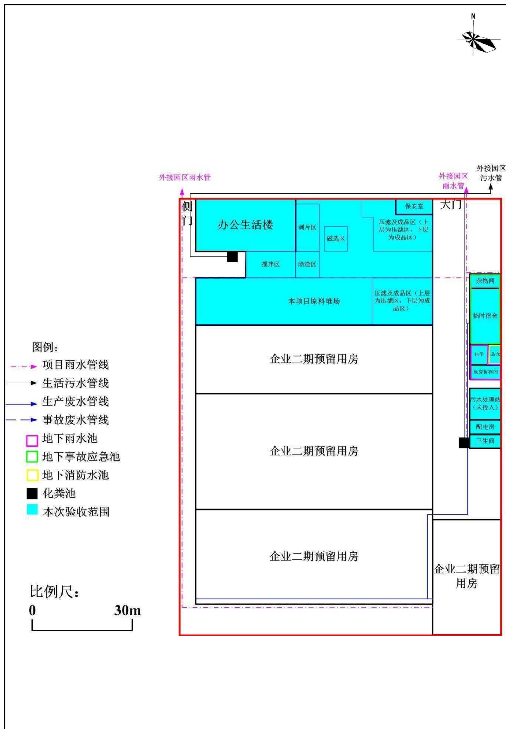
附图 5： 项目平面布置及雨污水管网图
