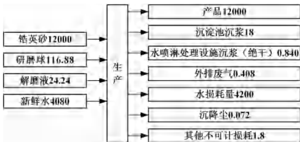
图2.1-3项目物料平衡图 (t/a)
