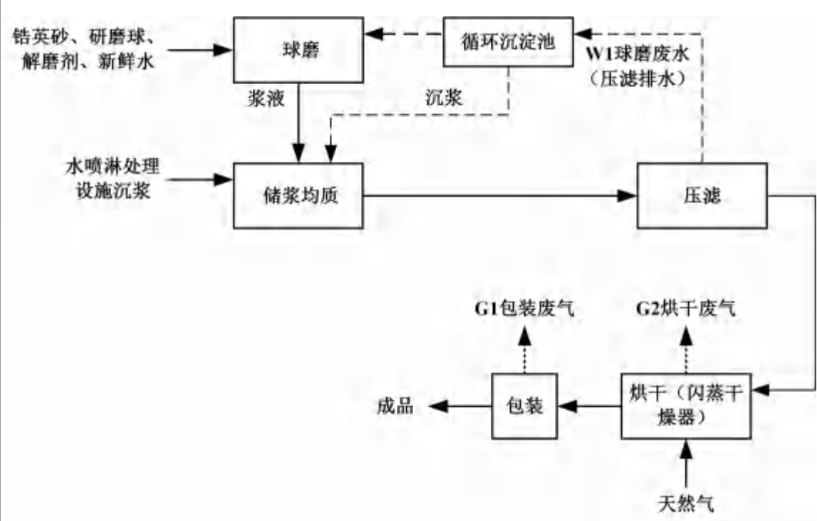
图 2.2-1 主体生产工艺及产污环节图
