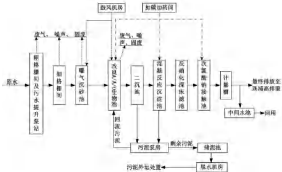
图 4.2-2 长泰区银塘污水处理厂工艺流程框图
