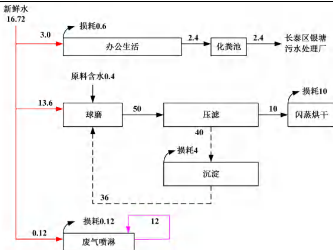
图 2.1-1 项目水平衡图 (m³/d)
